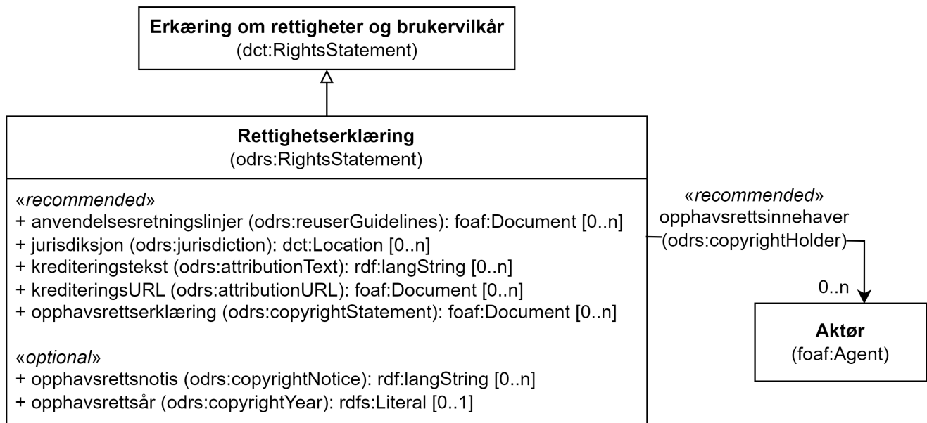
Figur 16. Klassen Rettighetserklæring og dens egenskaper.
