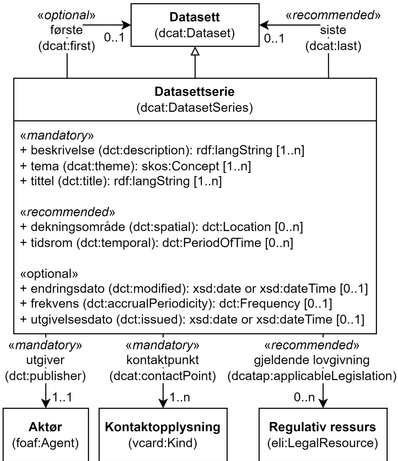
Figur 5. Klassen Datasettserie og klassene den refererer til.
