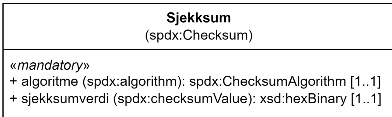
Figur 17. Klassen Sjekksum og dens egenskaper.
