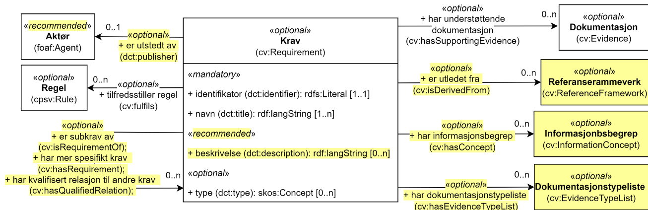
Figur 27. Klassen Krav (cv:Requirement) og klassene den refererer til.
