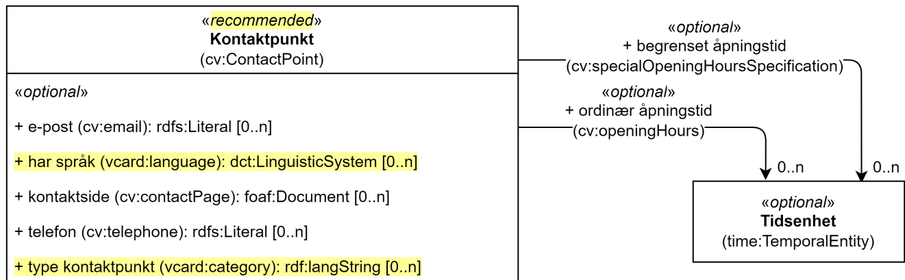
Figur 26. Klassen Kontaktpunkt (cv:ContactPoint) og klassen den refererer til.
