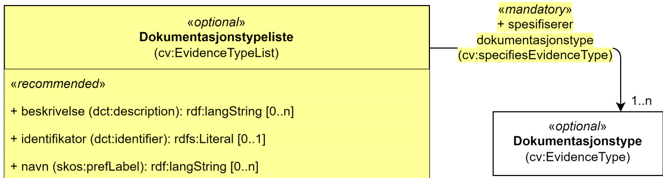
Figur 20. Klassen Dokumentasjonstypeliste (cv:EvidenceTypeList) og klassen den refererer til.
