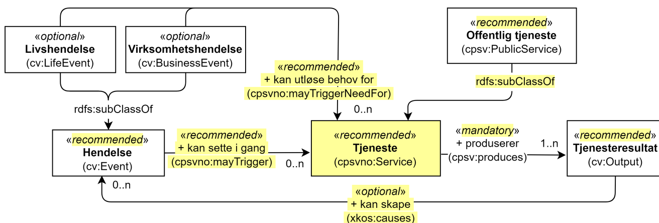
Figur 6. Klasser og egenskaper for beskrivelse av en tjenestekjede.
