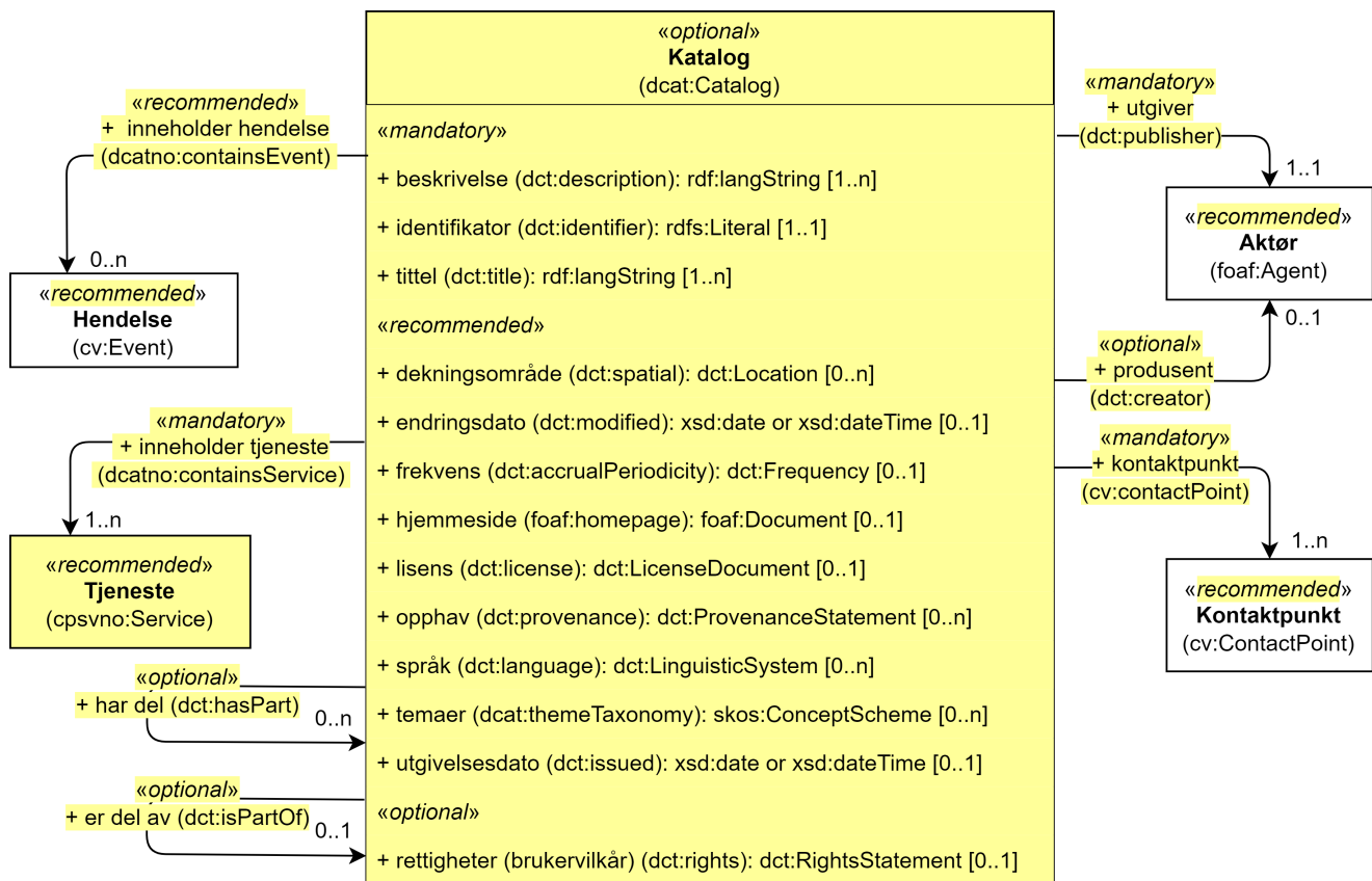
Figur 25. Klassen Katalog (dcat:Catalog) og klassene den refererer til.
