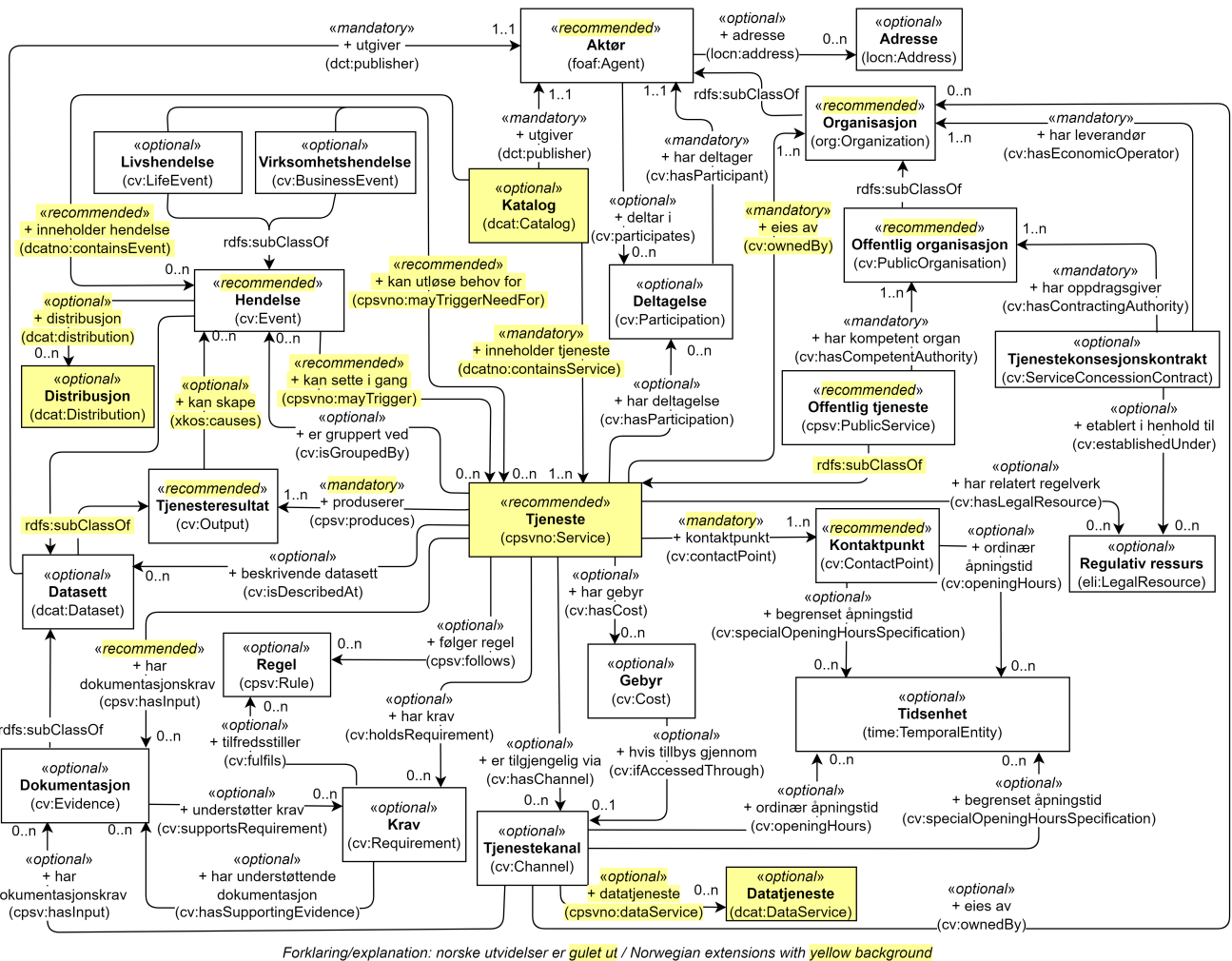
Figur 3. Forenklet modell for tjeneste- og hendelsesbeskrivelser.
