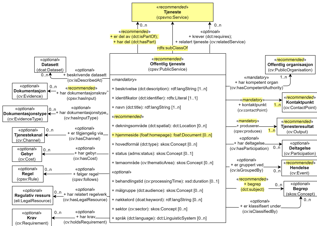
Figur 31. Klassen Offentlig tjeneste (cpsv:PublicService) og klassene den refererer til.
