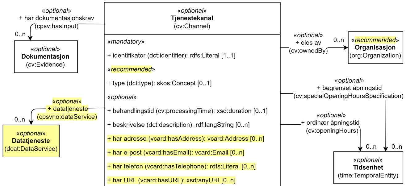
Figur 41. Klassen Tjenestekanal (cv:Channel) og klassene den refererer til.
