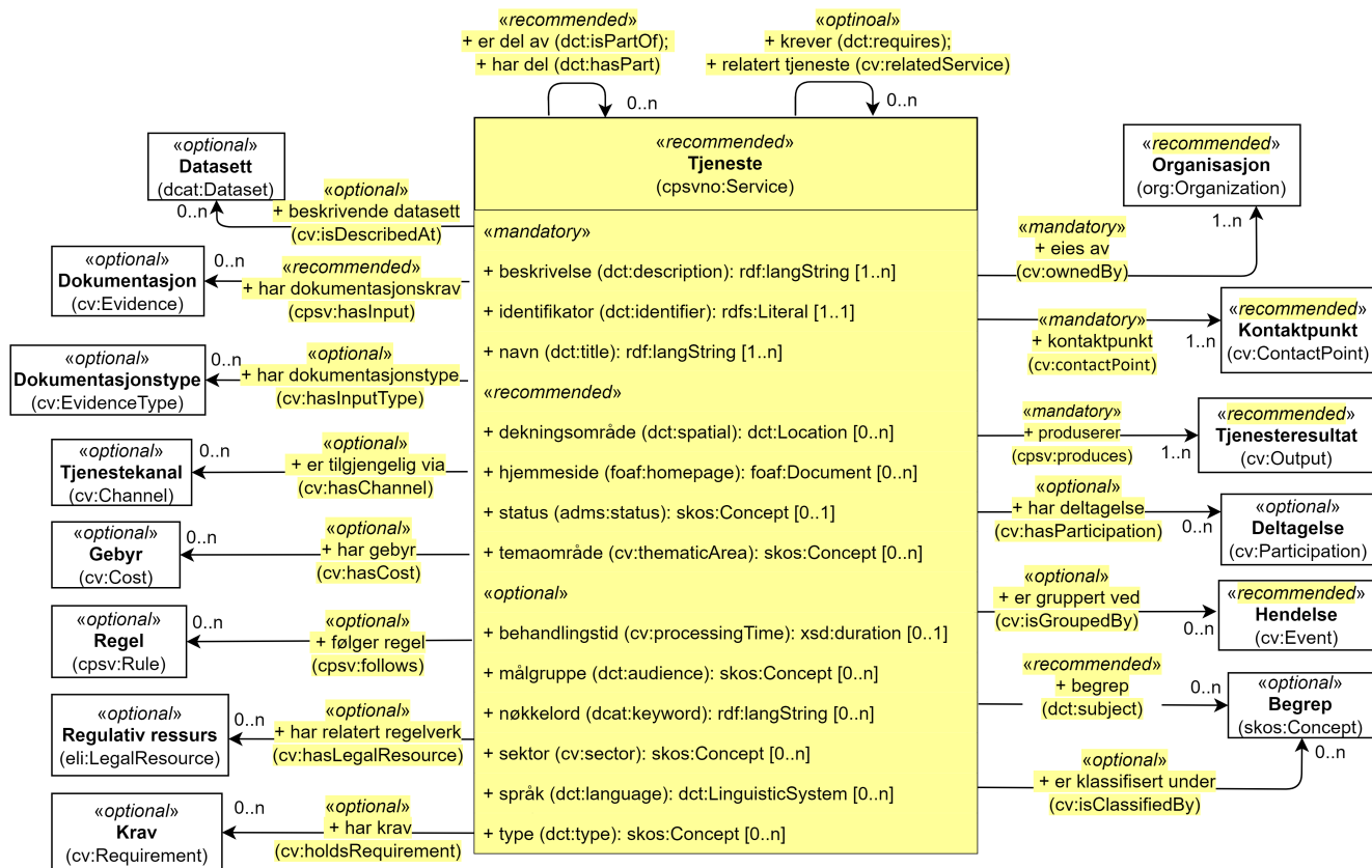
Figur 40. Klassen Tjeneste (cpsvno:Service) og klassene den refererer til.
