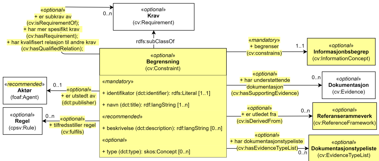
Figur 15. Klassen Begrensning (cv:Constraint) og klassene den refererer til.
