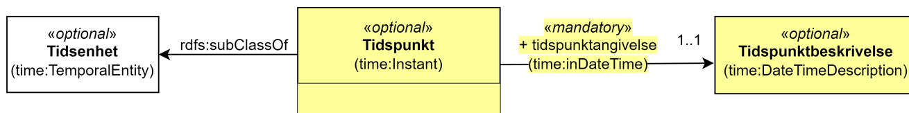
Figur 37. Klassen Tidspunkt (time:Instant) og klassene den refererer til.
