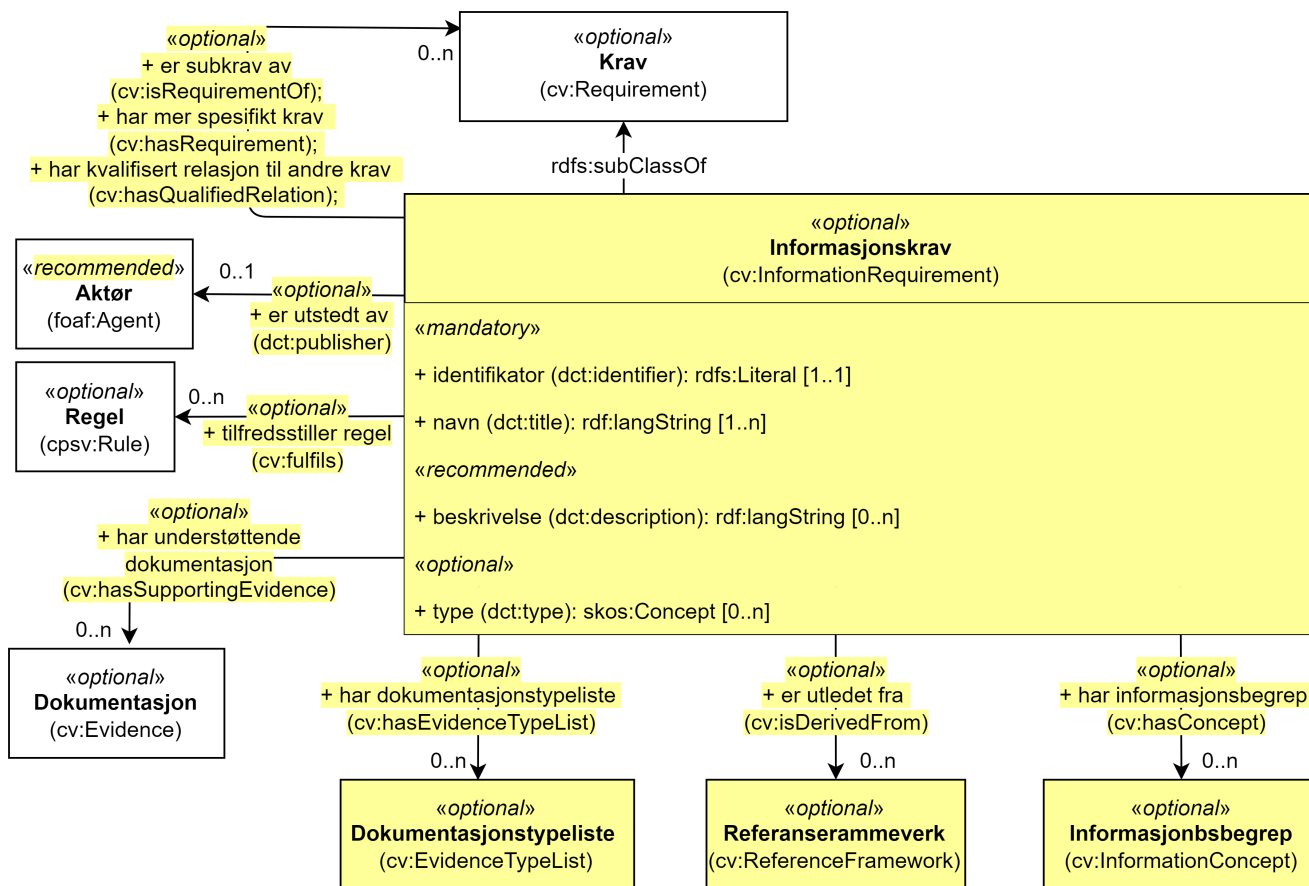
Figur 24. Klassen Informasjonskrav (cv:InformationRequirement) og klassene den refererer til.
