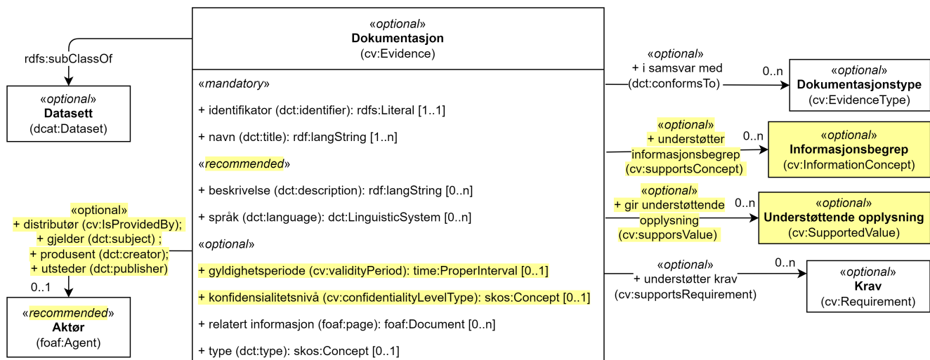
Figur 18. Klassen Dokumentasjon (cv:Evidence) og klassene den refererer til.
